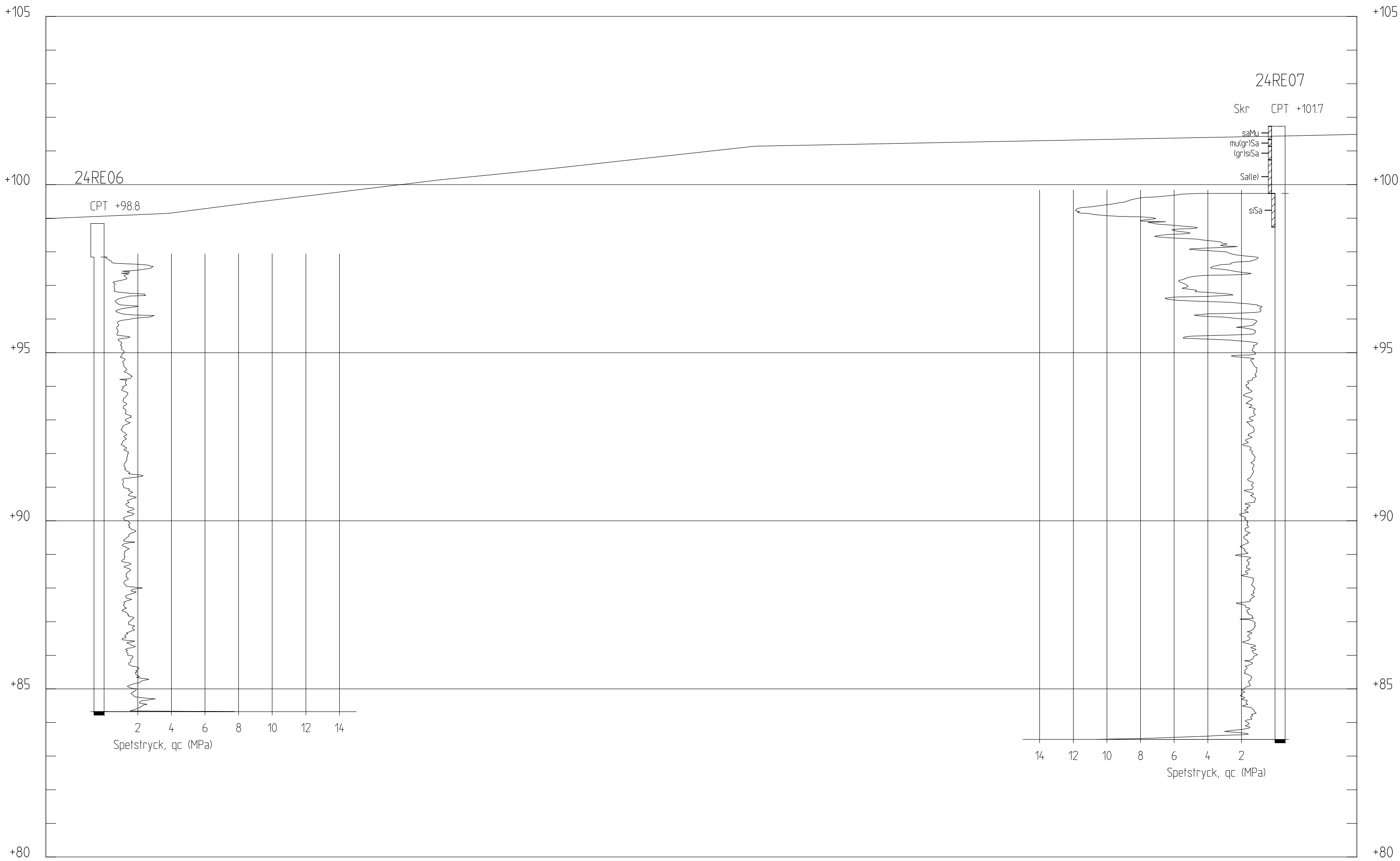
SEKTION C-C 1: 100
